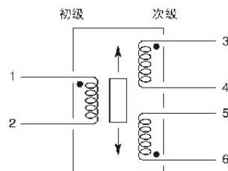
将(4)连接至(5)会产生差动输出
